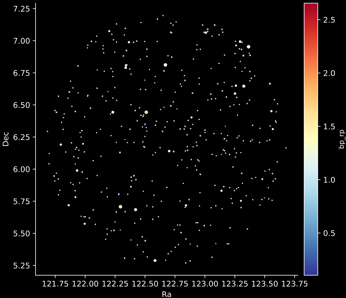
GALAH DR4 Field: [6679] Stars: 408
