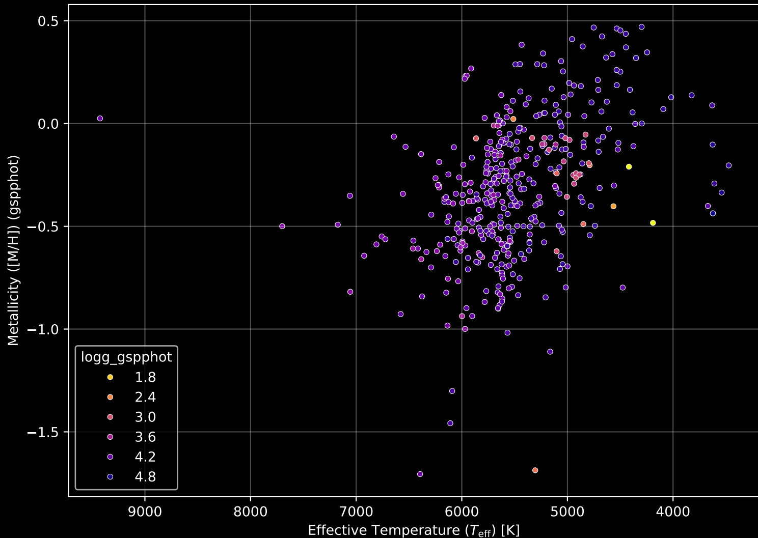
GALAH DR4 Field: [6679] Stellar Population Parameters (n= 408)
